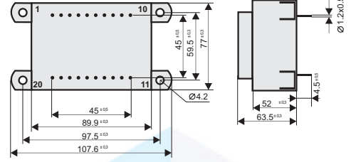
Pin Görüntüsü / Pin view Ölçüler mm'dir. / Dimension in mm.
