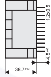
Pin Görüntüsü / Pin view Ölçüler mm'dir. / Dimension in mm.
