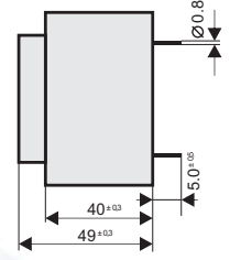
Pin Görüntüsü / Pin view Ölçüler mm'dir. / Dimension in mm.
