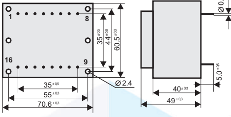
Pin Görüntüsü / Pin view Ölçüler mm'dir. / Dimension in mm.
