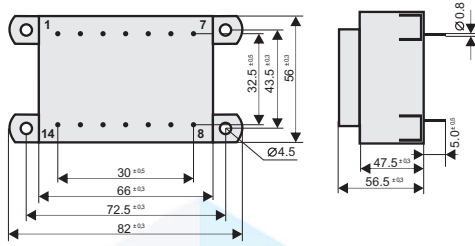
Pin Görüntüsü / Pin view Ölçüler mm'dir. / Dimension in mm.
