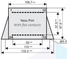
Pin Görüntüsü / Pin view Ölçüler mm'dir. / Dimension in mm.
