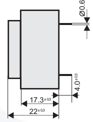
Pin Görüntüsü / Pin view Ölçüler mm'dir. / Dimension in mm.
