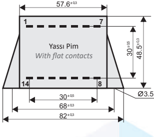
Pin Görüntüsü / Pin view Ölçüler mm'dir. / Dimension in mm.
