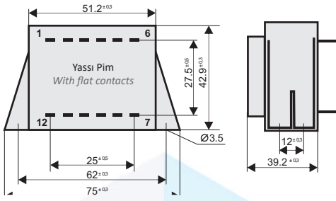
Pin Görüntüsü / Pin view Ölçüler mm'dir. / Dimension in mm.
