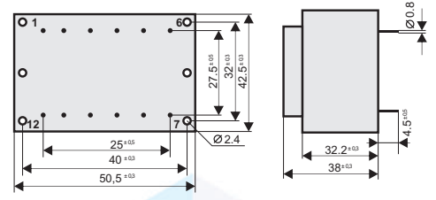
Pin Görüntüsü / Pin view Ölçüler mm'dir. / Dimension in mm.
