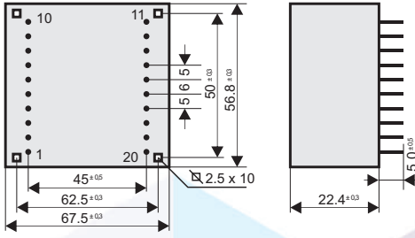
Pin Görüntüsü / Pin view Ölçüler mm'dir. / Dimension in mm.
