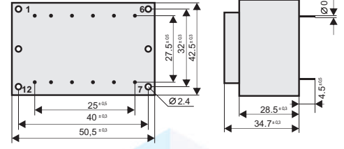
Pin Görüntüsü / Pin view Ölçüler mm'dir. / Dimension in mm.
