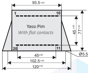
Pin Görüntüsü / Pin view Ölçüler mm'dir. / Dimension in mm.
