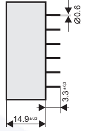
Pin Görüntüsü / Pin view Ölçüler mm'dir. / Dimension in mm.
