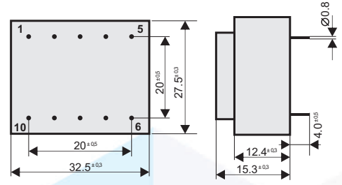
Pin Görüntüsü / Pin view Ölçüler mm'dir. / Dimension in mm.
