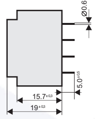
Pin Görüntüsü / Pin view Ölçüler mm'dir. / Dimension in mm.
