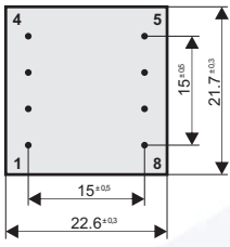
Pin Görüntüsü / Pin view Ölçüler mm'dir. / Dimension in mm.
